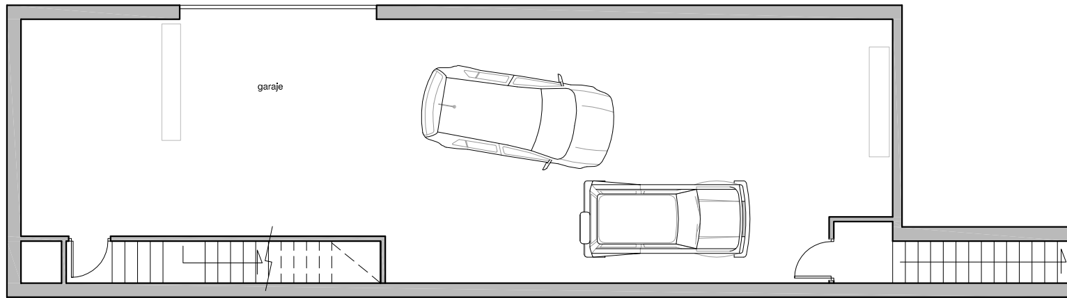
Planta sótano
