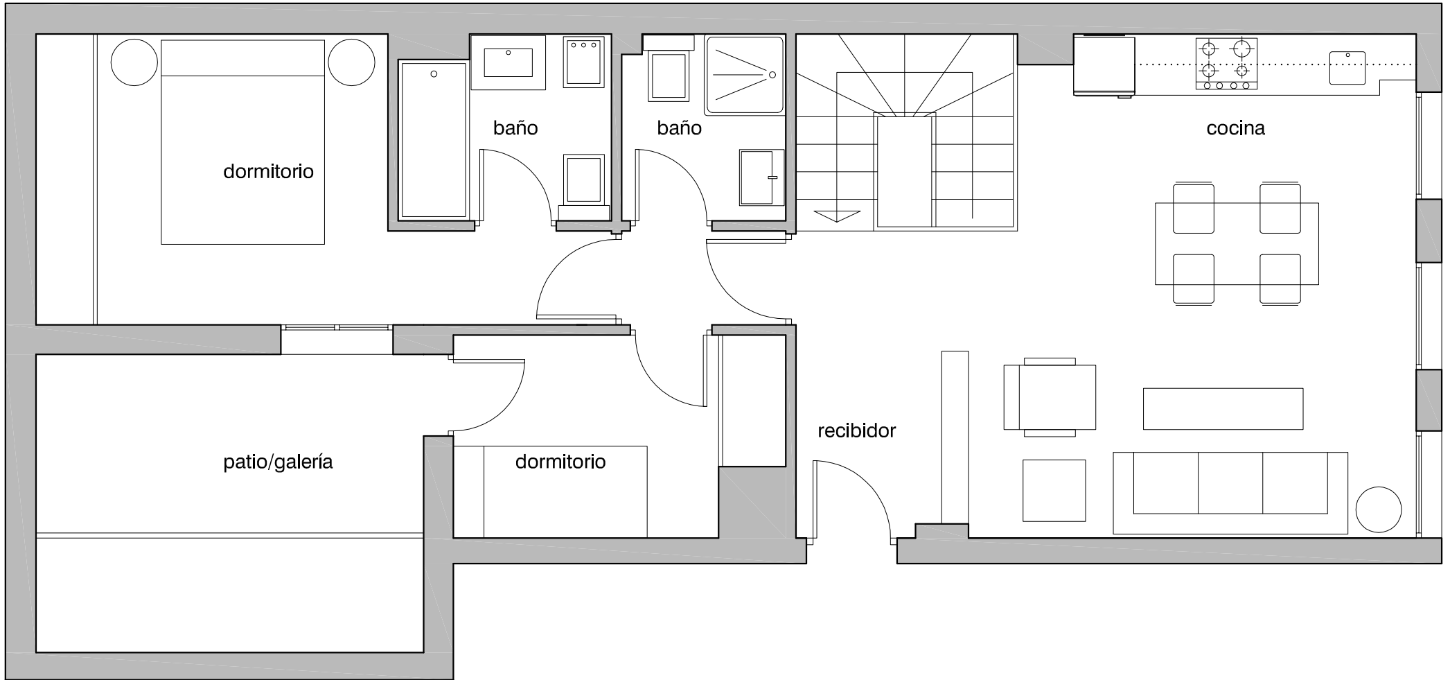
Planta baja
