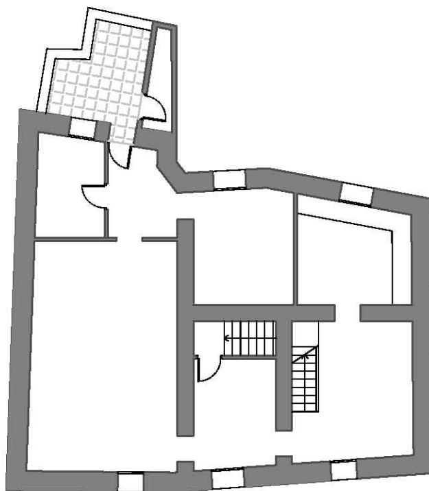
PLANTA PIS 1
