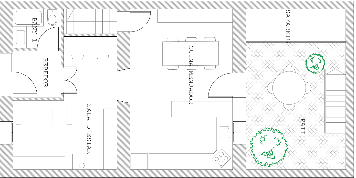
PLANTA BAIXA
