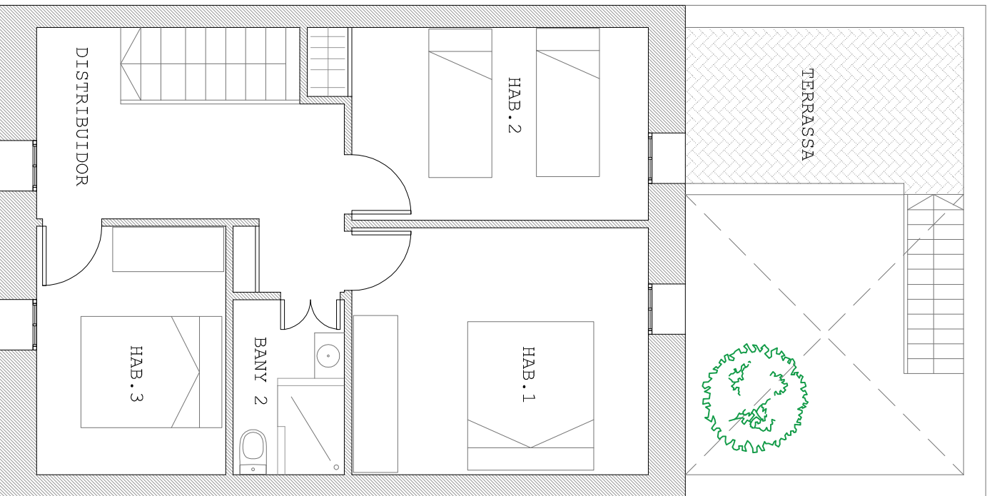
PLANTA PRIMERA
