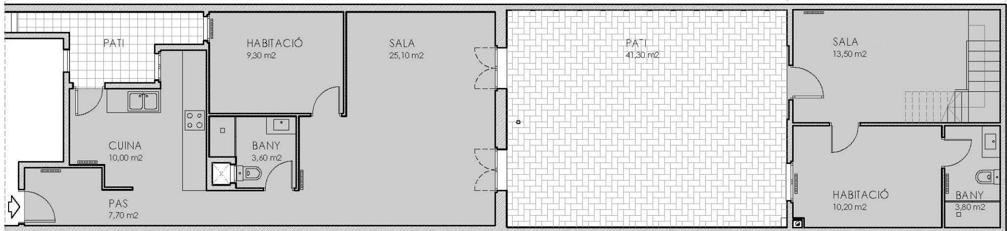
PLANTA BAIXA
