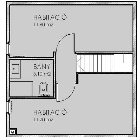
PLANTA PRIMERA
