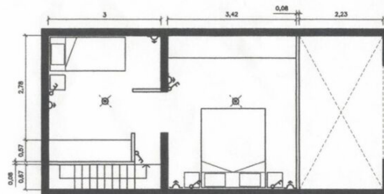
PROPUESTA ELECTRICA
