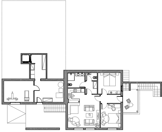
PLANTA -1
