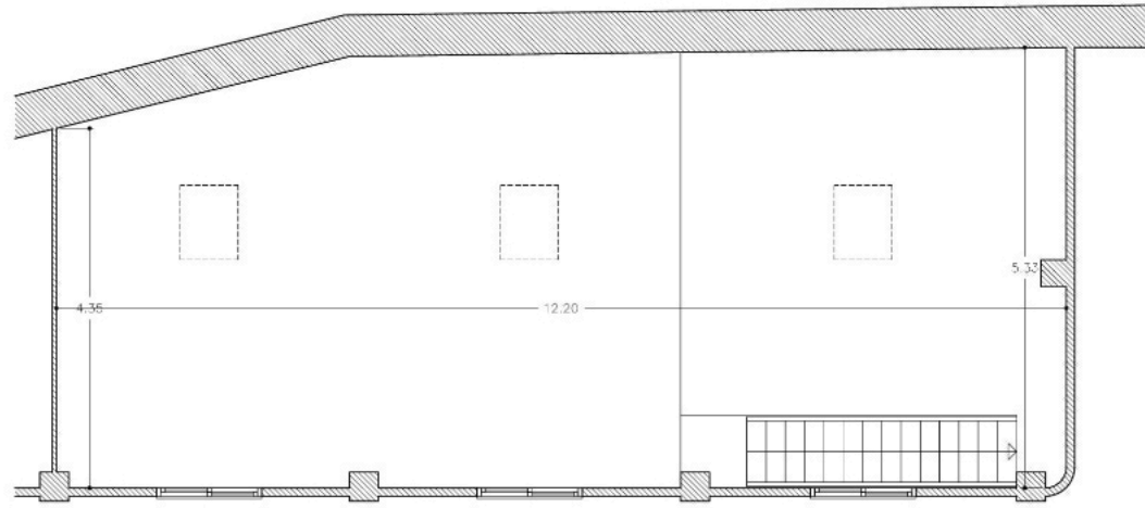
PLANTA PRIMERA
