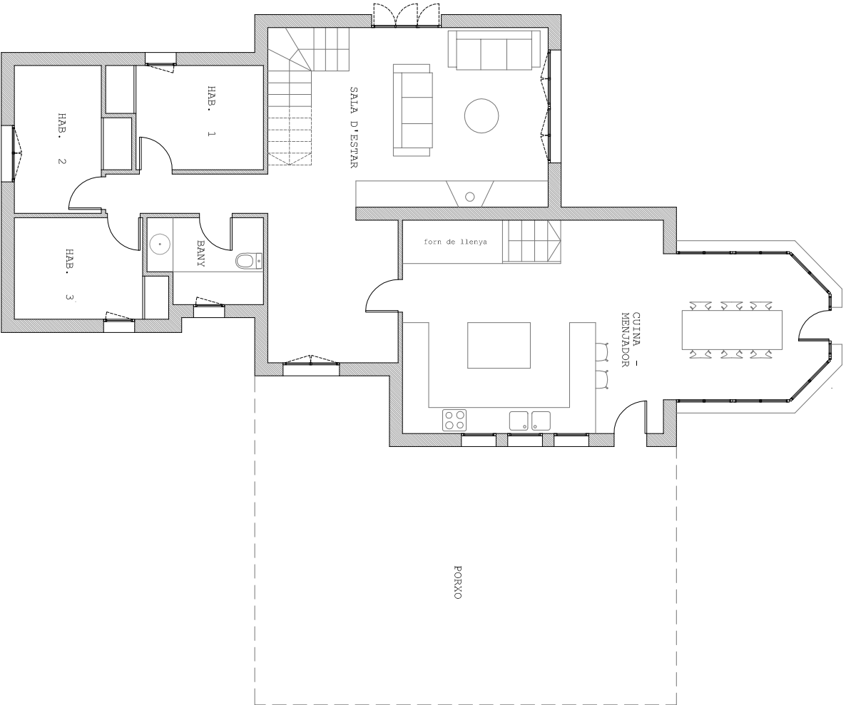
PLANTA BAIXA
