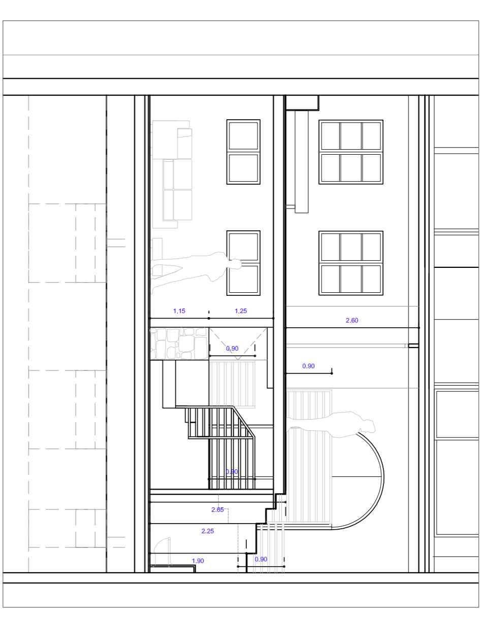
HABITATGE 1. SECCIO ESCALA E 1:75
